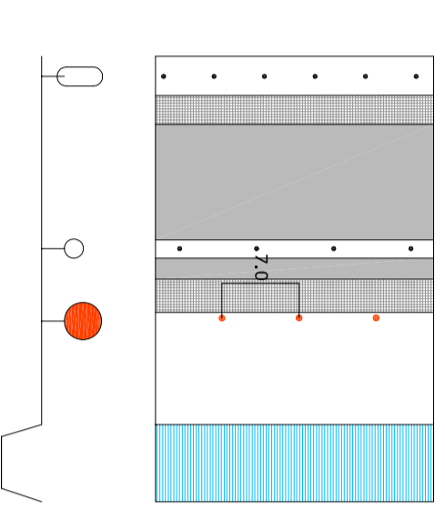
PLANTACIÓ EXISTENT I REPLANTACIÓ
